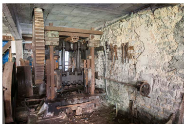
La presse. Phot. Jérôme Mongreville IVR43_20152501244NUC4A
