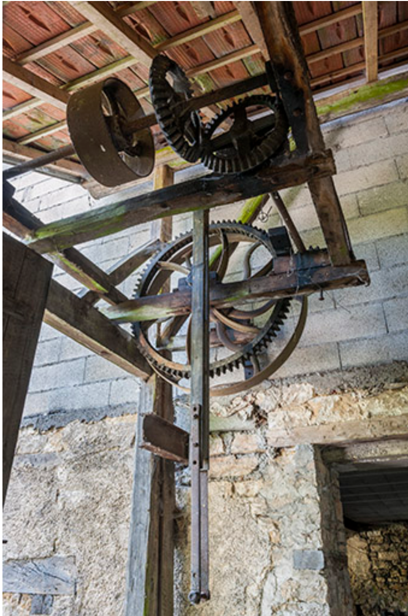
Bâtiment d'eau. Système de transmission des soufflets de la forge (disparus).
