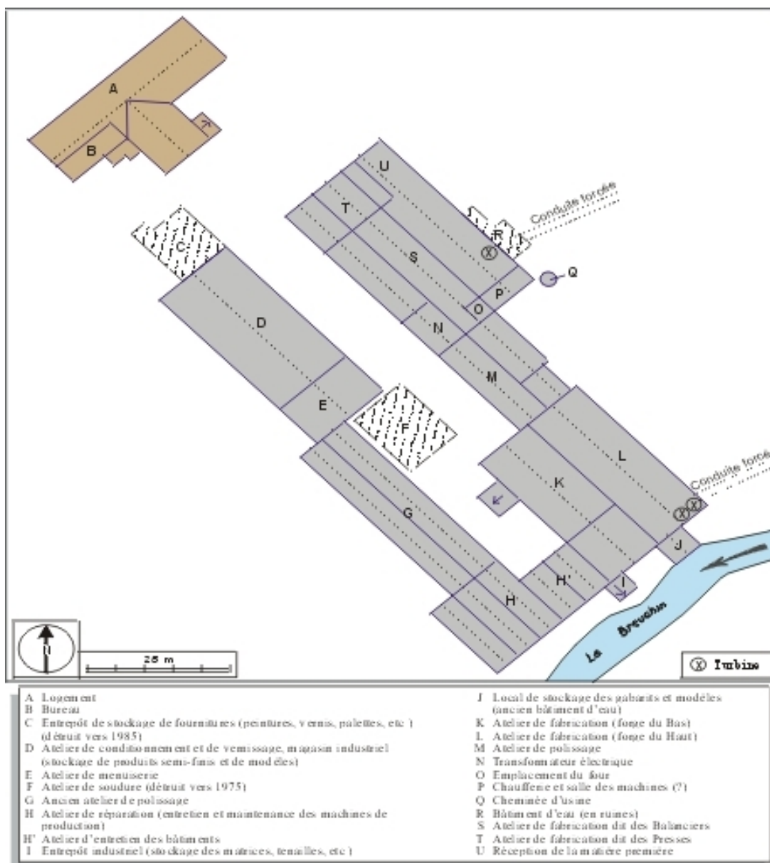
Plan-masse de l'usine. Extrait du plan cadastral, 2004, section AC, 1:1000 agrandi à 1:750.
