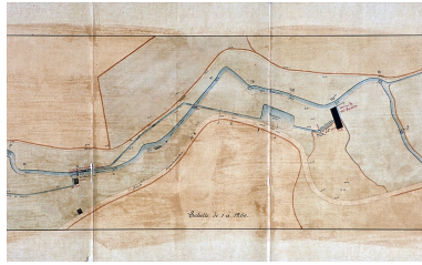
Projet de règlement de l'usine à faulx de Corravillers au sieur Clément Paxion. Plan des lieux. Phot. Jérôme Mongreville, Autr. Celler IVR43_20057000565NUCA
