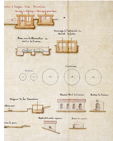
Projet de règlement de l'usine à faulx de Corravillers au sieur Clément Paxion. Plan des lieux [coupes et élévations]. Phot. Jérôme Mongreville, Autr. Celler IVR43_20057000567NUCA
