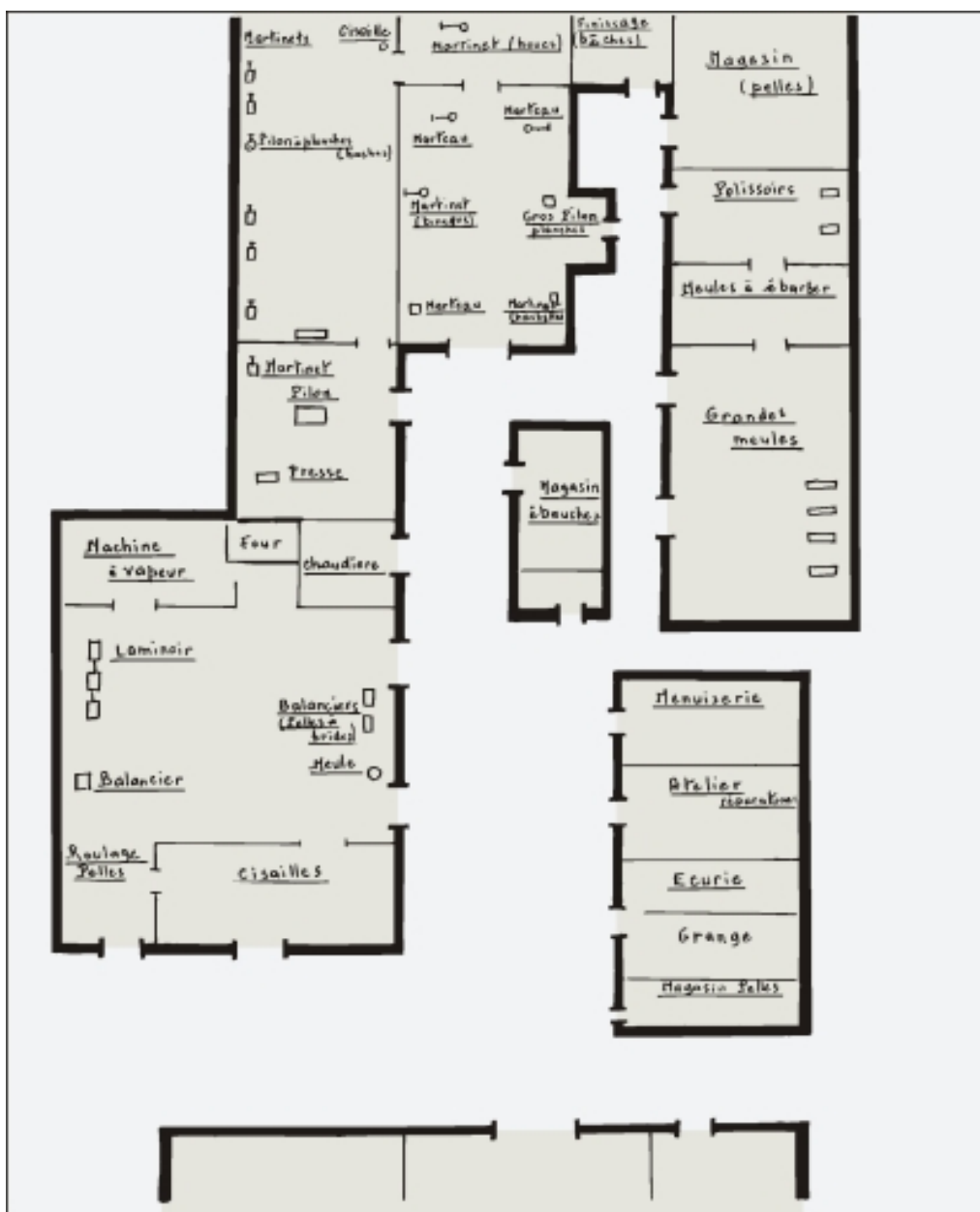
Schéma de localisation des machines en 1920.
