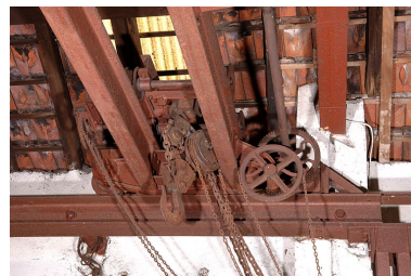
Atelier dit des Balanciers. Le palan du pont roulant. Phot. Jérôme Mongreville IVR43_20057000103NUCA
