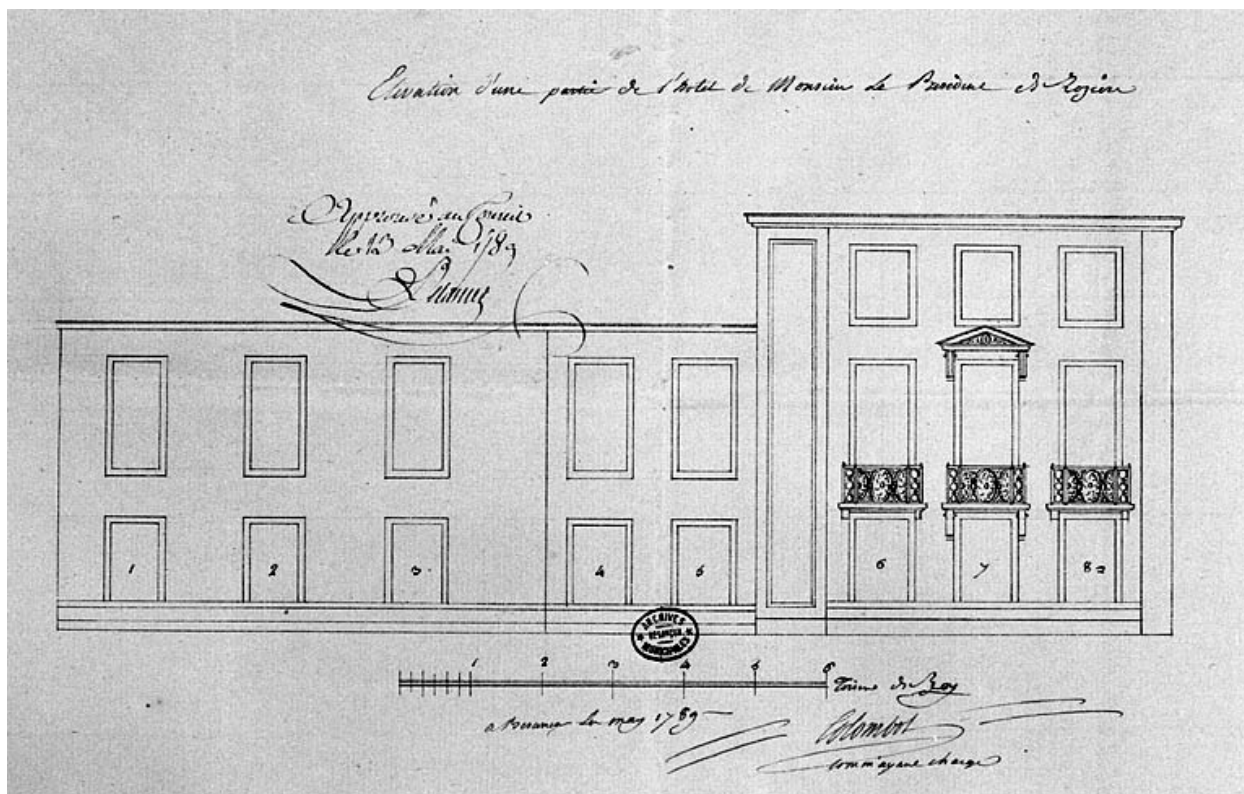
Elévation de la façade sur rue. Dessin à la plume, premier mai 1789
