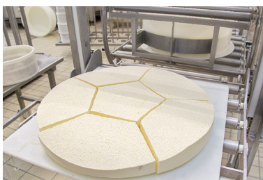
Fabrication du morbier : pain de caillé découpé en épaisseur. Phot. Sonia Dourlot IVR43_20142500770NUC2A
