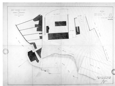
Haut fourneau de Dole. Terrain et dépendances. Phot. Yves Sancey, Autr. Jules Decoursière IVR43_19903901027X
