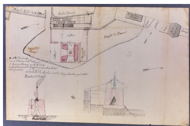
Haut fourneau de la Lampinette à Dole. Plan de détail. Phot. Jérôme Mongreville IVR43_20013900306XA
