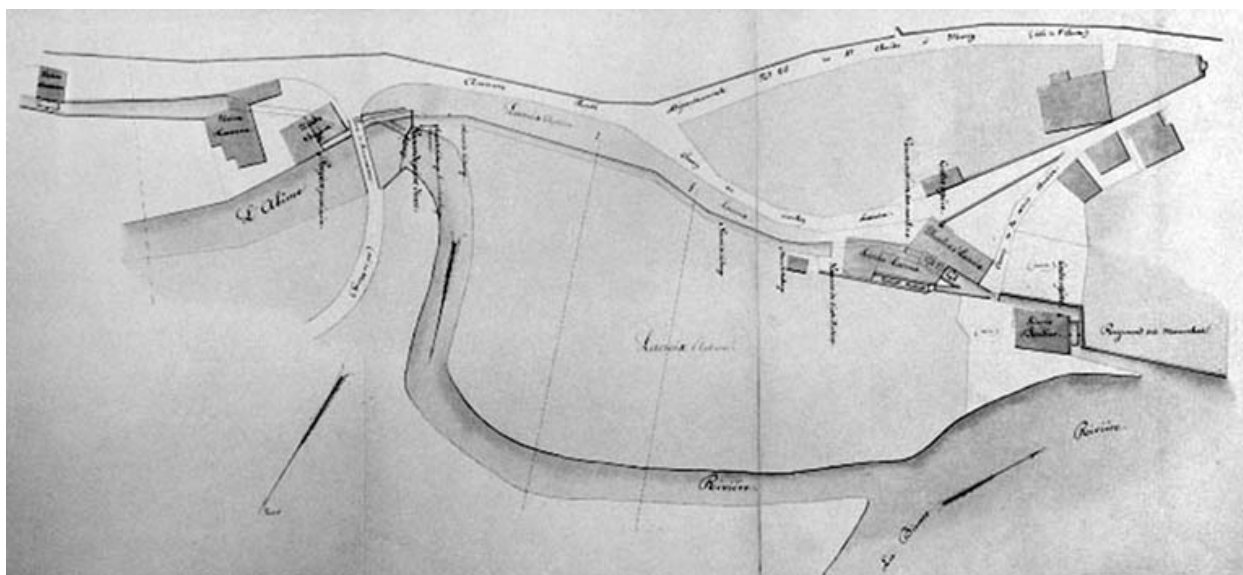
Réglementation de l'usine du Sr Lacroix Antoine. Plan des lieux et dessins de détail.
