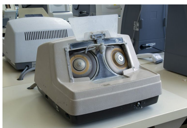
Ecole professionnelle dite Ecole nationale d'Optique puis lycée polyvalent Victor Bérard, Morez : meuleuse manuelle Essilor MD2.
