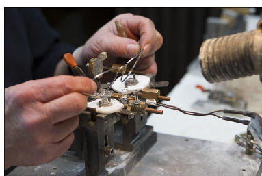
Usine Gouverneur-Audigier, Morez : soudage sur la machine à souder Himmel. Phot. Yves Sancey IVR43_20103900321NUC2A
