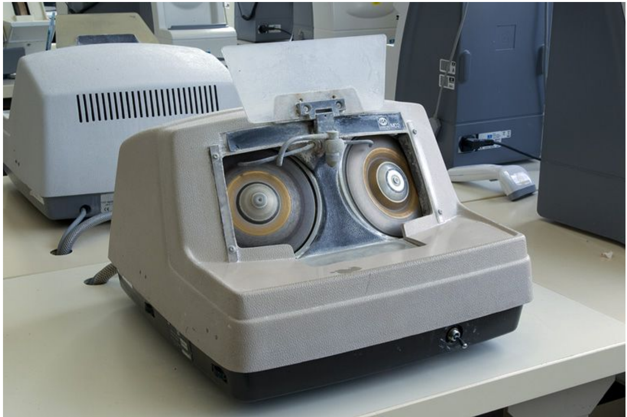
Ecole professionnelle dite Ecole nationale d'Optique puis lycée polyvalent Victor Bérard, Morez : meuleuse manuelle Essilor MD2.
