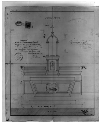
Production : Maître-Autel [projet d'autel-tabernacle-dais d'exposition]. Phot. Jérôme Mongreville, Autr. Célard IVR43_19933900373V
