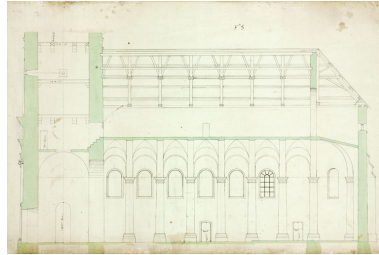
[Coupe longitudinale de l'église]. S.d. [31 mai 1788]. Phot. Jérôme Mongreville, Autr. Anatoile Amoudru IVR43_20112502603NUC4A
