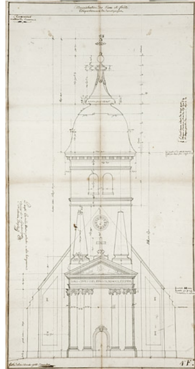
[Elévation de la façade de l'église]. S.d. [31 mai 1788]. Phot. Jérôme Mongreville, Autr. Anatoile Amoudru IVR43_20112502606NUC4A
