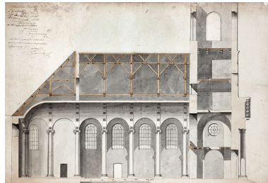
[Coupe longitudinale de l'église]. S.d. [1789]. Phot. Jérôme Mongreville, Autr. Claude-Joseph-Alexandre Bertrand IVR43_20112502602NUC4A
