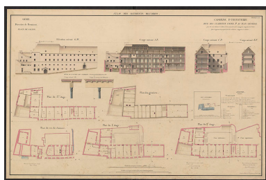
Génie. Direction de Besançon. Place de Salins. Caserne d'infanterie dite des Clarisses, 1851. Phot. Jean-Pierre Compas IVR43_20223901214NUC4A
