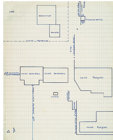
[Plan-masse et de situation partiel de l'usine Farque dressé à l'occasion de l'installation d'une citerne de gaz], [1964]. Phot. Jérôme Mongreville, Autr. auteur inconnu IVR43_20132500531NUC4A
