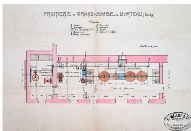
Fruitière de Grand-Combe de Morteau (Doubs) [plan de l'installation], 1913 ? Phot. Jérôme Mongreville, Autr. R. Wallut et Cie IVR43_20192500048NUC4A
