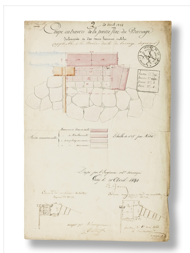
Coupe en travers de la partie fixe du Barrage. [Détail des maçonneries]. 1844 Phot. Thierry Kuntz
