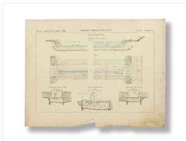
Barrage mobile d'Heuilley. Plan, coupe et élévation. 1886. Phot. Thierry Kuntz IVR26_20172100140NUC4A
