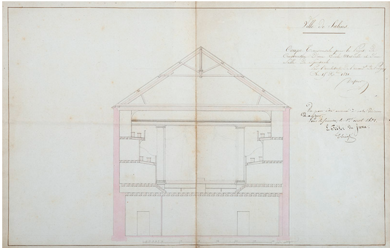
Coupe transversale pour le projet de construction d'une école mutuelle et d'une salle de spectacle, 1831.
