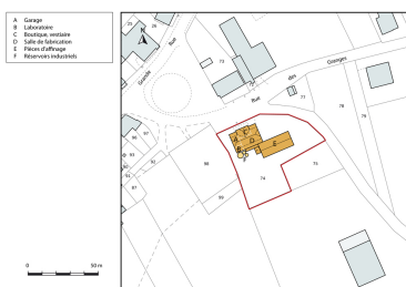
Plan-masse et de situation, section AB. Dess. Mathias Papigny IVR43_20142501928NUDA
