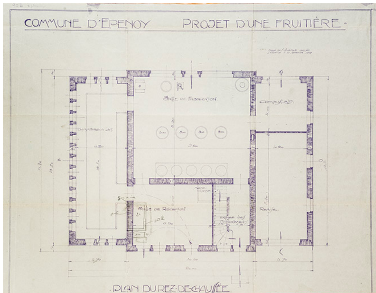
Commune d'Epenoy. Projet d'une fruitière. Plan du rez-de-chaussée, 1929.
