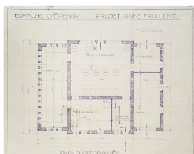
Commune d'Epenoy. Projet d'une fromagerie. Plan du rez-de-chaussée, 1929. Phot. Jérôme Mongreville IVR43_20152500568NUC4A
