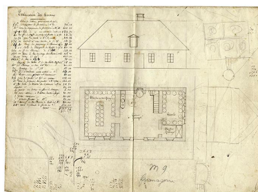
[Projet de fromagerie : plan et élévation], 1859. Autr. auteur inconnu IVR43_20182500040NUC4A
