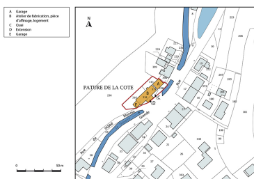
Plan-masse et de situation. Extrait du plan cadastral, 2017, section AC, 1/1 000. Dess. Mathias Papigny IVR43_20172501249NUDA
