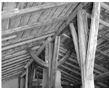
Charpente, colonne sous faîtage et contrefiche. Phot. Jérôme Mongreville IVR43_20013900470X
