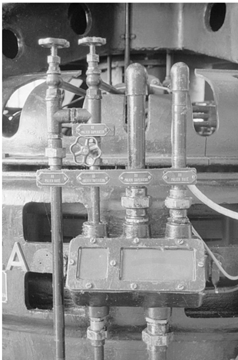
Alternateur ASEA : détail des conduits de graissage.
