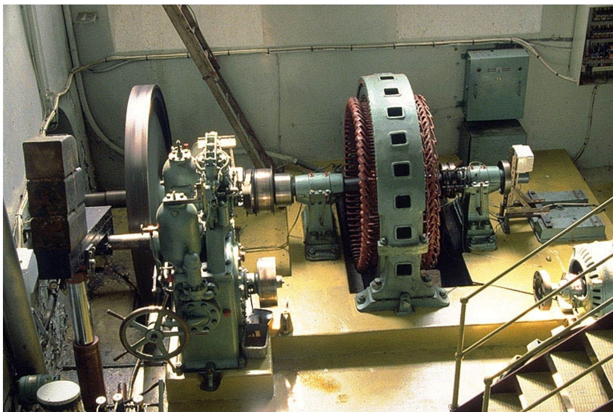
Intérieur de la salle des machines (D).Arbre de couche d'une turbine Francis, régulateur et alternateur de 1914.
