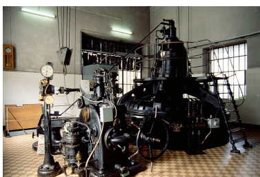
Intérieur de la salle des machines (C). Commande d'admission d'eau de la turbine Kaplan et alternateur ASEA. Phot. Laurent Poupard IVR43_19903900482ZA
