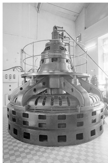
Alternateur ASEA. Phot. Laurent Poupard
