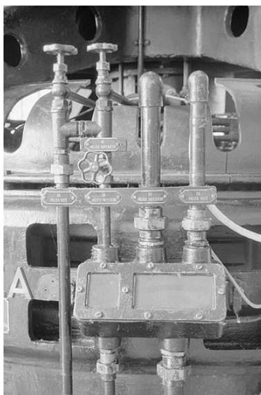
Alternateur ASEA : détail des conduits de graissage. Phot. Laurent Poupard IVR43_19903900485Z
