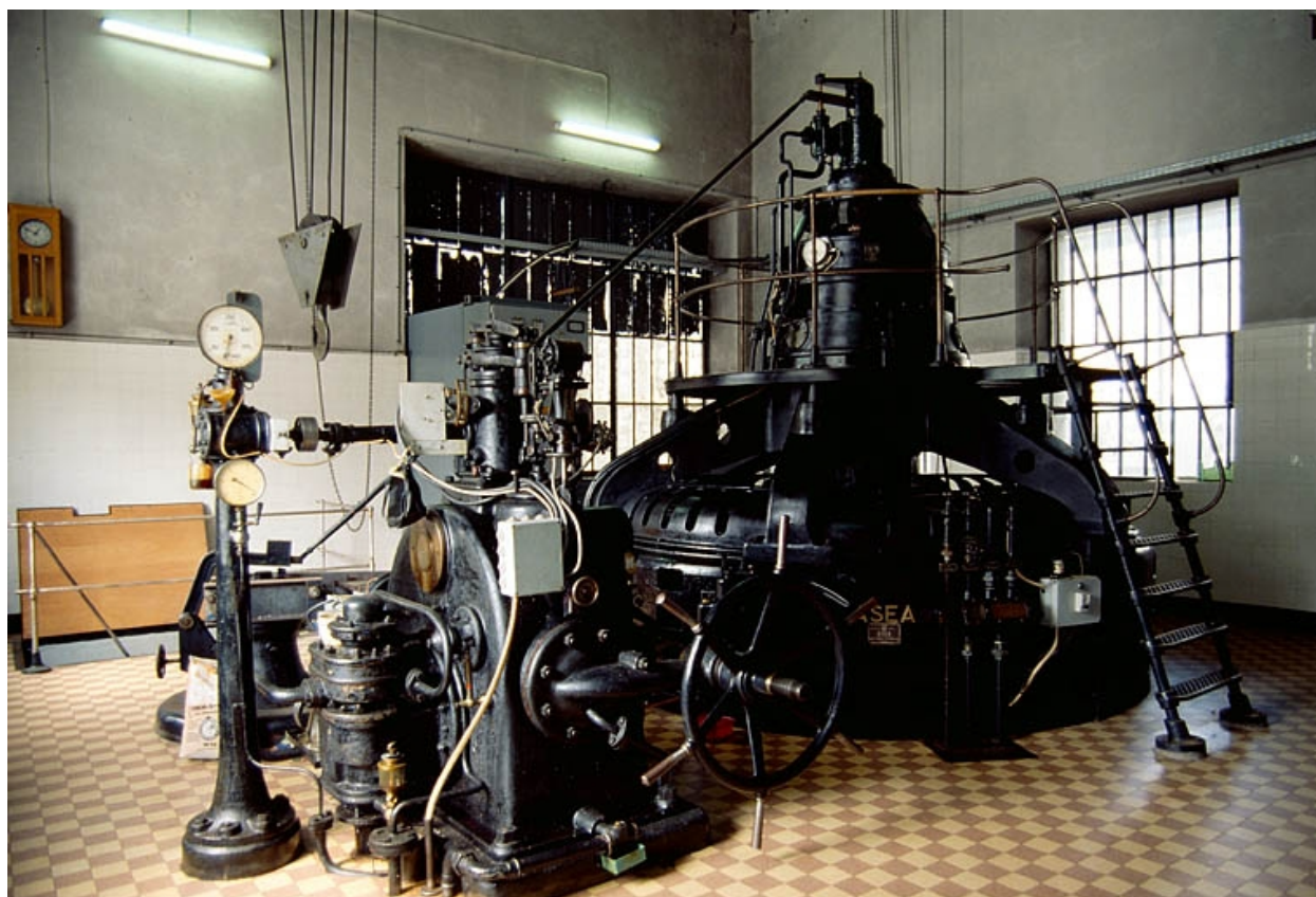
Intérieur de la salle des machines (C).Commande d'admission d'eau de la turbine Kaplan et alternateur ASEA.
