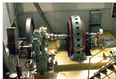
Intérieur de la salle des machines (D).Arbre de couche d'une turbine Francis, régulateur et alternateur de 1914. Phot. Laurent Poupard IVR43_19903900486ZA
