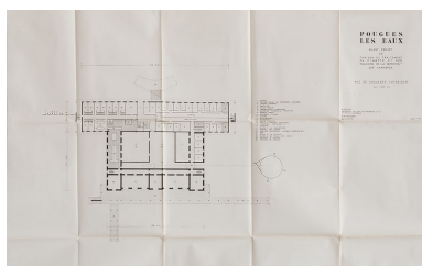
Avant-projet d'une maison du diabète dans le parc thermal, plan du rez-de-chaussée inférieur (1960). Phot. Pierre-Marie Barbe-Richaud, Autr. Raymond Gleize, Autr. André Noël Coquet IVR26_20205800142NUC2A
