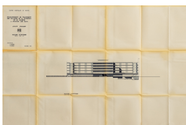
Avant-projet d'une maison du diabète aux Chailloux, façade d'entrée (1965). Autr. Pierre-Marie Barbe-Richaud, Autr. Armand Inconnu, Autr. André Noël Coquet, Autr. Pierre Coquet IVR26_20205800386NUC4A
