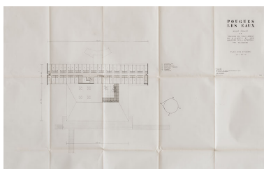
Avant-projet d'une maison du diabète dans le parc thermal, plan des étages (1960). Phot. Pierre-Marie Barbe-Richaud, Autr. Raymond Gleize, Autr. André Noël Coquet IVR26_20205800143NUC2A
