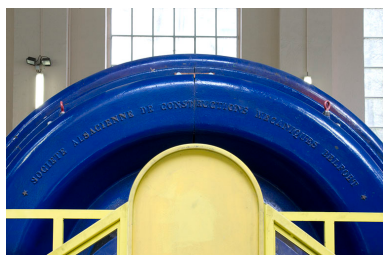
Groupe n° 2 : inscription sur le capot de l'alternateur. Phot. Yves Sancey IVR43_20122502135NUC2A
