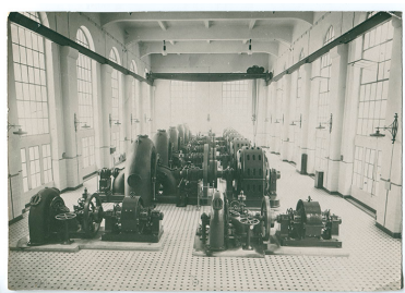
[Intérieur de la centrale], [1909 ?]. Autr. auteur inconnu IVR43_20172500017NUC4A
