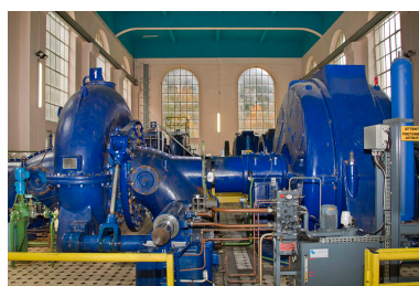
Groupe n° 1 : face avant. Phot. Yves Sancey IVR43_20122502120NUC2A
