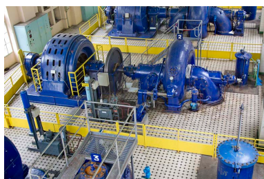
Groupe n° 2 : face arrière. Phot. Yves Sancey IVR43_20122502144NUC2A
