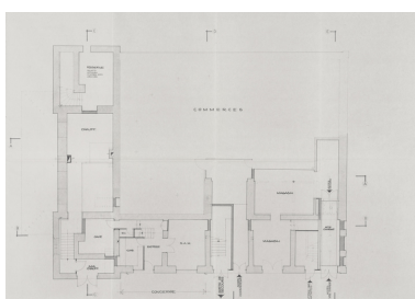
Ville d'Autun. Théâtre municipal. Place du Champ de Mars. Projet de rénovation. 7706 13. Niveau sous-sol. S.d. [1978 ?]. Phot. Pierre-Marie Barbe- Richaud, Autr. Jean- Pierre Caudin, Autr. Didier Grillot IVR26_20257100214NUC4A
