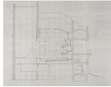
Ville d'Autun. Théâtre municipal. Place du Champ de Mars. Projet de rénovation. 7706 20. Coupe long. AA sur salle. Février 1978. Phot. Pierre-Marie Barbe- Richaud, Autr. Jean- Pierre Caudin, Autr. Didier Grillot IVR26_20257100209NUC4A
