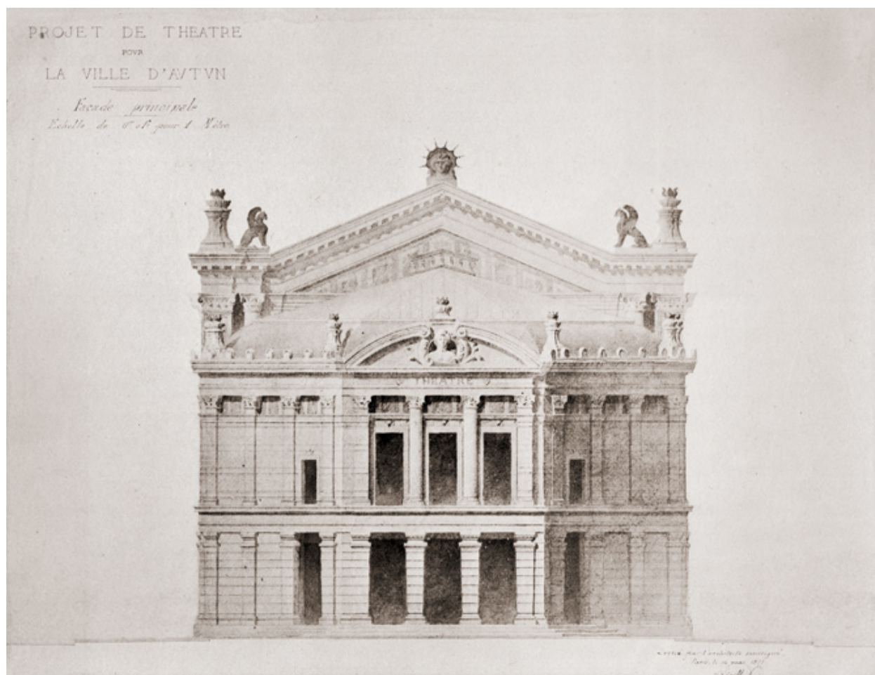
Projet de théâtre pour la ville d'Autun. Façade principale. 14 mai 1877.
