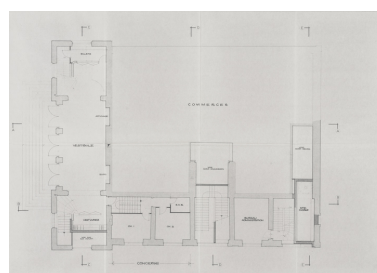
Ville d'Autun. Théâtre municipal. Place du Champ de Mars. Projet de rénovation. 7706 14. Niveau vestibule. S.d. [1978 ?]. Phot. Pierre-Marie Barbe- Richaud, Autr. Jean- Pierre Caudin, Autr. Didier Grillot IVR26_20257100213NUC4A
