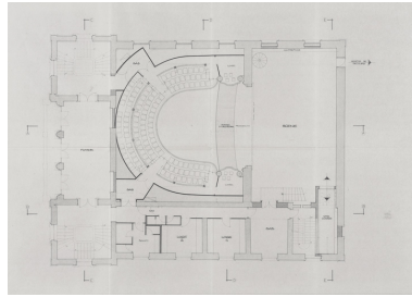
Ville d'Autun. Théâtre municipal. Place du Champ de Mars. Projet de rénovation. 7706 16. Niveau 1ère galerie. S.d. [1978 ?]. Phot. Pierre-Marie Barbe- Richaud, Autr. Jean- Pierre Caudin, Autr. Didier Grillot IVR26_20257100211NUC4A
