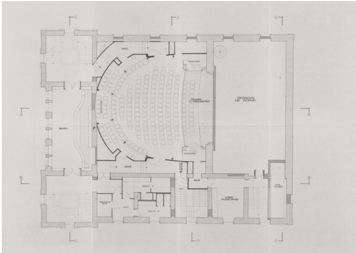
Ville d'Autun. Théâtre municipal. Place du Champ de Mars. Projet de rénovation. 7706 15. Niveau parterre. S.d. [1978 ?].
