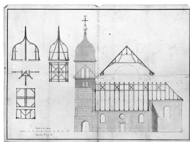
Plan, coupe et élévations de l'église.
