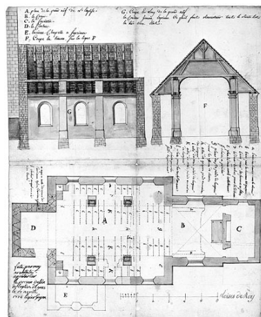
Plan et coupes de l'église.
