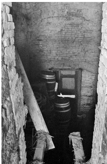
Intérieur du 1er four, depuis la porte d'enfournement. La voûte du foyer a été supprimée. Phot. Laurent Poupard IVR43_19883900534Z
