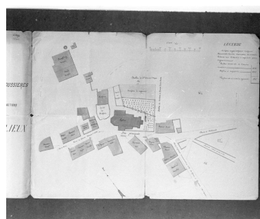
Commune des Moussières. Agrandissement du cimetière. Plan des lieux. Phot. Jérôme Mongreville, Phot. Boisson IVR43_19943901382X
