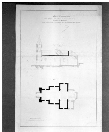
Projet de construction d'un clocher, d'un choeur et d'une sacristie à l'église des Moussières [coupe longitudinale et plan]. Phot. Jérôme Mongreville, Phot. Auguste Comoy IVR43_19943901392X
