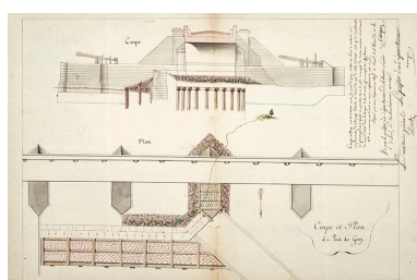
Coupe et plan sur la 3e arche du pont de Gray (1802). Phot. Jérôme Mongreville, Autr. Claude Ignace Lingée IVR43_20197000414NUC4A
