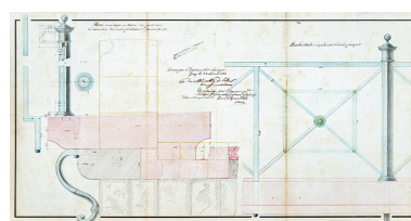
Balustrade remplaçant l'ancien parapet, 1842. Phot. Jérôme Mongreville, Autr. Mathy de La Tour ou de La Tour Mathy IVR43_20197000411NUC4A
