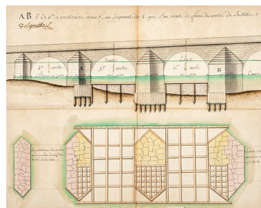
Plan et élévation des 5e et 6e arches du pont de Gray (entre 1735 et 1742). Phot. Jérôme Mongreville, Autr. Jean-François de Légouthail IVR43_20197000417NUC4A
