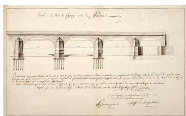
Dessin d'une partie du pont (1802). Phot. Jérôme Mongreville, Autr. Claude Ignace Lingée IVR43_20197000413NUC4A
