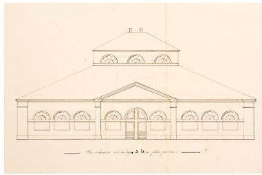
Plan de détail de l'usine de Varigney [façade antérieure de l'atelier du haut fourneau]. Phot. Jérôme Mongreville, Autr. Bernard IVR43_20077000055NUCA
