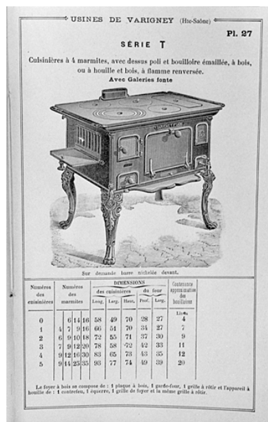
Catalogue des productions : cuisinière à 4 marmites. Phot. Bernard Lardière IVR43_19807000097Z
