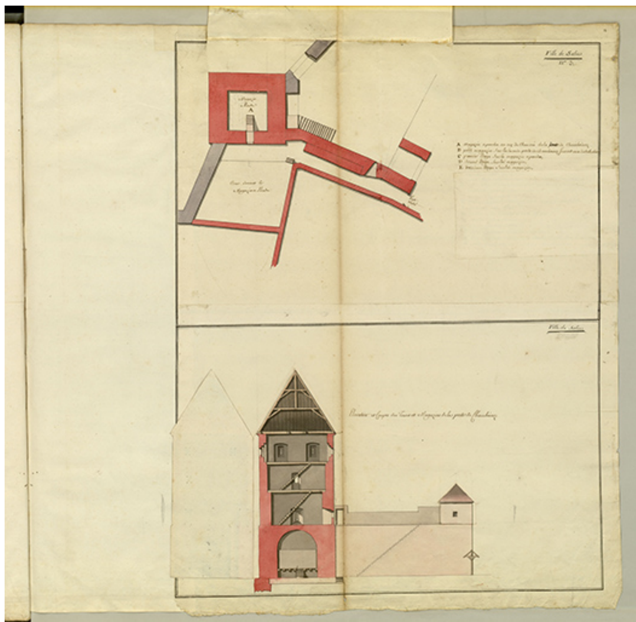
Folio 14. Ville de Salins. Tour et magasin à poudre de la porte de Chamboinoz. N°3. Plan, coupe et élévation. Magasin à poudre, 1756.
