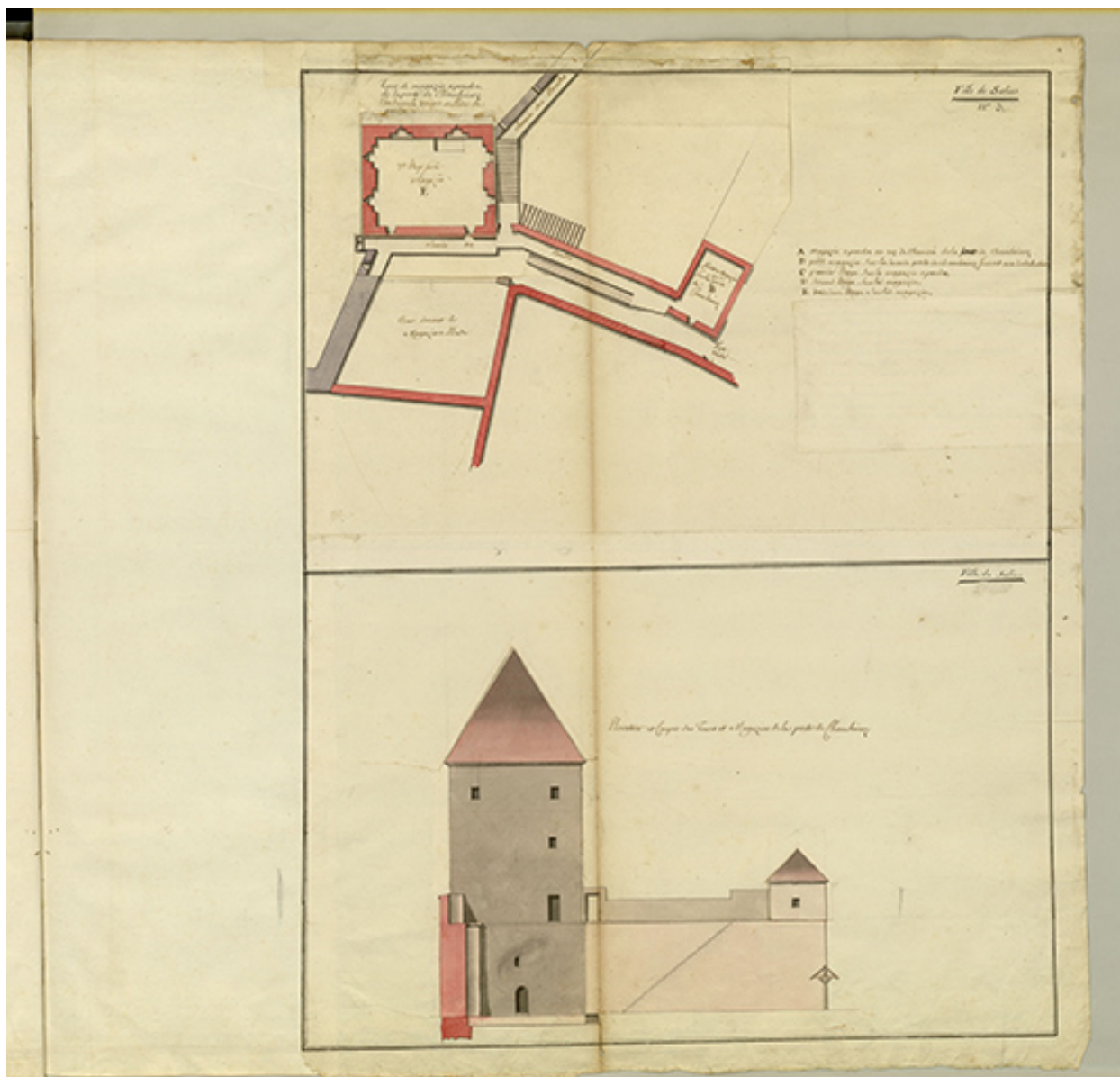
Folio 14. Ville de Salins. Tour et magasin à poudre de la porte de Chamboinoz. N°3. Plan, coupe et élévation. Troisième étage sur le magasin, 1756.
