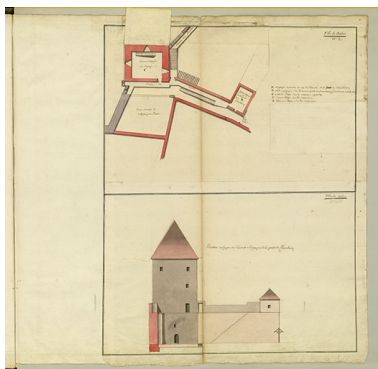
Folio 14. Ville de Salins. Tour et magasin à poudre de la porte de Chamboinoz. N°3. Plan, coupe et élévation. Premier étage sur le magasin, 1756.
