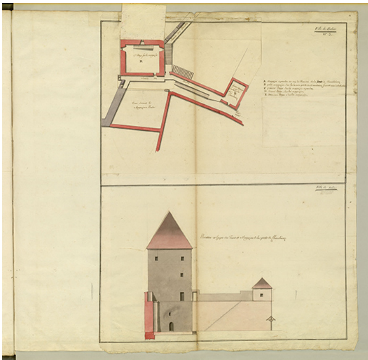
Folio 14. Ville de Salins. Tour et magasin à poudre de la porte de Chamboinoz. N°3. Plan, coupe et élévation. Deuxième étage sur le magasin, 1756.
