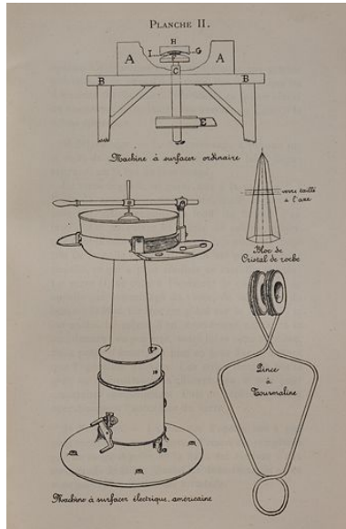
Machine à surfacer ordinaire [et] Machine à surfacer électrique américaine, 1913.
