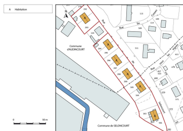
Plan-masse et de situation. Dess. Mathias Papigny IVR43_20132502558NUDA
