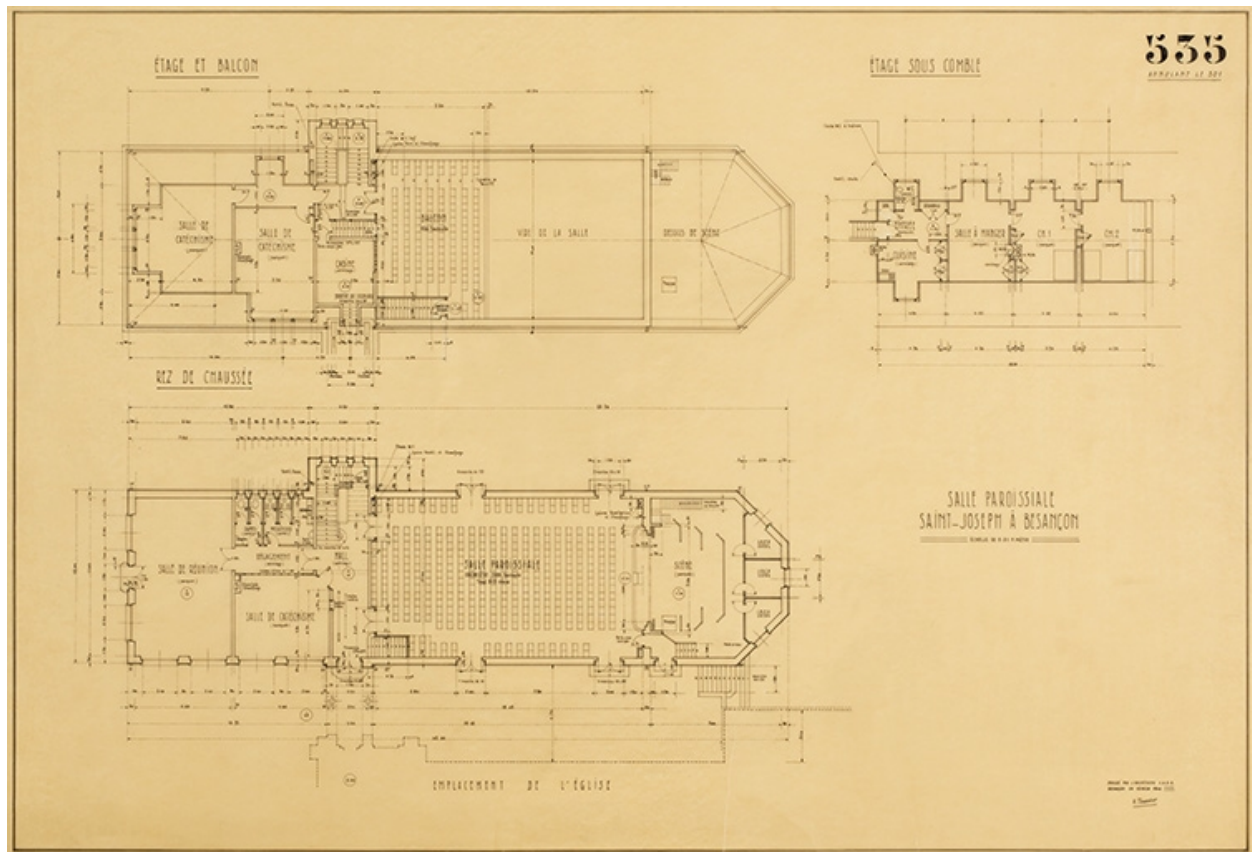
Salle paroissiale Saint-Joseph à Besançon : plan du rez-de-chaussée, de l'étage et balcon et de l'étage sous comble. Février 1946.
