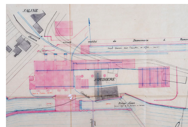
[Plan de la Soudière], 1891. Phot. Jérôme Mongreville IVR43_20182500087NUC4A
