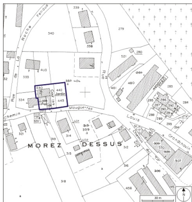
Plan-masse et de situation. Extrait du plan cadastral, 1980, section AI, échelle 1:1000. Dess. André Céréza IVR43_20093900312NUDA
