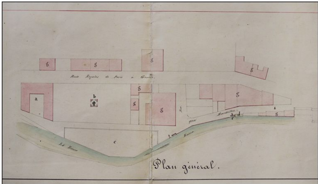
Plan et profils d'un mur de soutènement pour le quai Mandrillon et d'un lavoir à établir dans la ville de Morez : dessin (plume, lavis), 10 mai 1842, échelles diverses.
