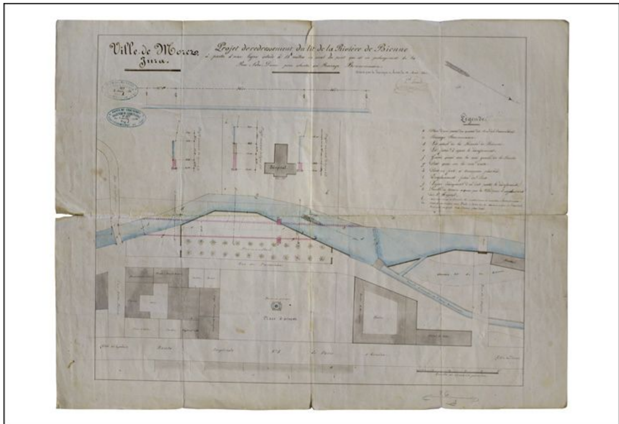
Projet de redressement du lit de la rivière de Bienne [...] : dessin (plume, lavis), 30 avril 1860, échelle 1:500.
