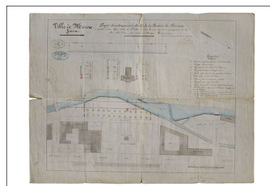
Projet de redressement du lit de la rivière de Bienne [...] : dessin (plume, lavis), 30 avril 1860, échelle 1:500. Phot. Yves Sancey, Phot. Vital Ponard IVR43_20103900090NUC2A
