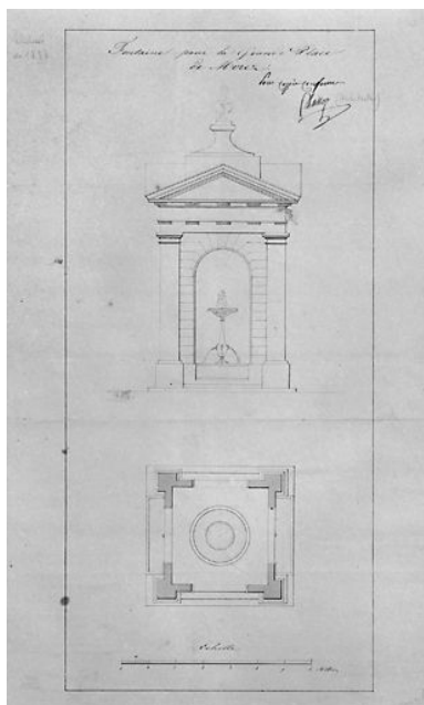
Fontaine pour la Grande Place de Morez [plan et élévation] : dessin (plume, lavis), s.d. [vers 1836], échelle approximative 1:70. Phot. Jérôme Mongreville, Phot. Claude-Marie Dalloz IVR43_19953900048X
