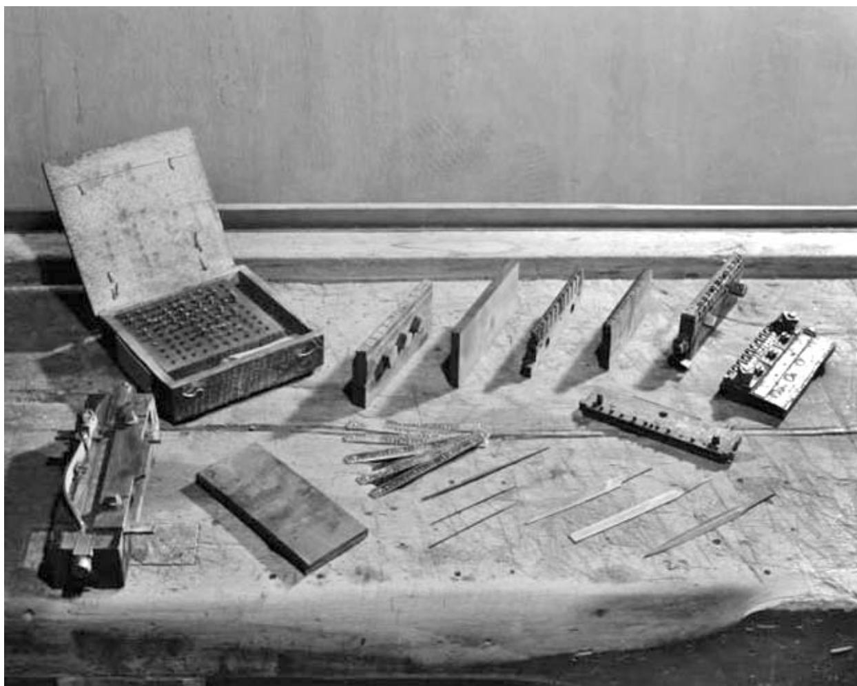
Poinçons à différents stades de fabrication.
