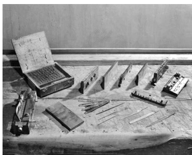
Poinçons à différents stades de fabrication. Phot. Yves Sancey IVR43_19913900770X
