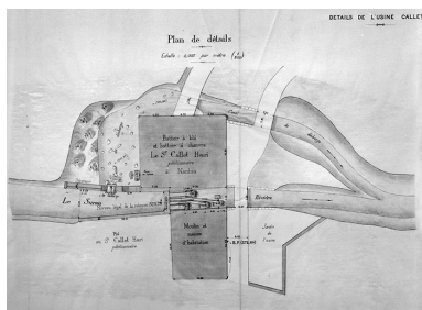
Réglement d'eau du Moulin des Prés appartenant à M. Callet Henri. Plans d'ensemble et de détails et profil en long. Phot. Jérôme Mongreville, Autr. NEPASUTILISERPernot (conducteur de travaux) IVR43_19943900454X
