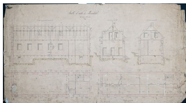
Salle d'asile du Rondelot. Plan, plume, encre, lavis, échelle 1/50, s.d. [fin 19e ou début 20e]. Phot. Jérôme Mongreville IVR43_20122501214NUC4A
