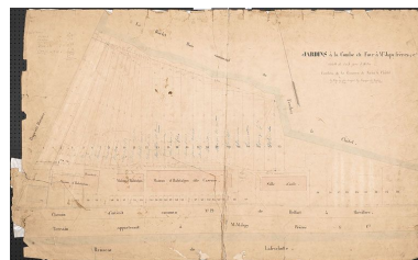
Jardins à la Combe du Four à MM. Japy Frères et Cie. Plan, plume, encre, lavis, échelle 1/200, s.d. [fin 19e ou début 20e]. Phot. Jérôme Mongreville IVR43_20122501182NUC4A
