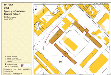
Plan-masse et de situation. Extrait du plan cadastral numérisé, section BV, échelle 1:1250. Dess. André Céréza IVR43_20123900011NUDA
