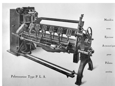
Pelotonneuse automatique type P.L.A. Phot. Yves Sancey IVR43_19953900127X
