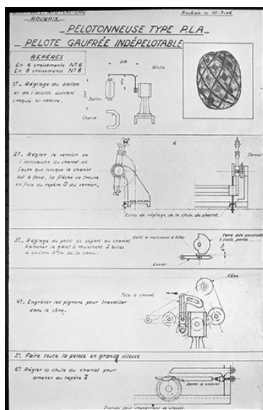
Pelotonneuse type P.L.A. Pelote gaufrée indépelotable [notice de réglage de la machine]. Phot. Yves Sancey IVR43_19953900128X
