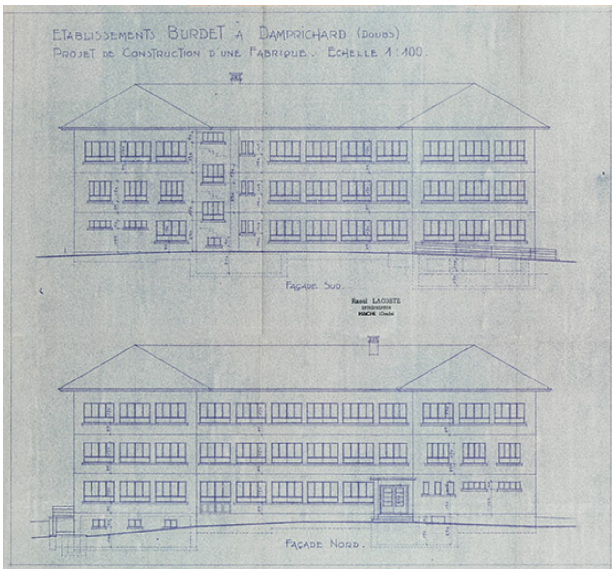
Établissements Burdet à Damprichard (Doubs). Projet de construction d'une fabrique [élévations sud et nord], [1951].
