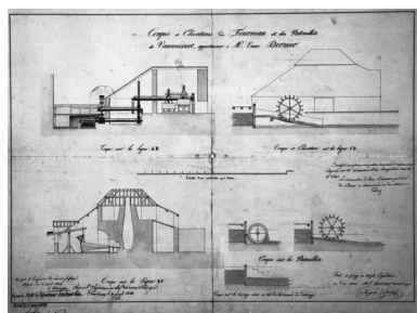
Coupes et élévations du fourneau et des patouillets de Vauconcourt, appartenant à Mme veuve Dornier. Phot. Yves Sancey, Autr. Auguste Sirodot IVR43_19877000085X
