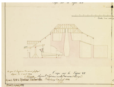
Coupes et élévations du fourneau et des patouillets de Vauconcourt [coupe du haut fourneau]. Phot. Jérôme Mongreville, Autr. Auguste Sirodot IVR43_20097000030NUC2A
