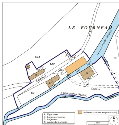
Plan-masse et de situation. Extrait du plan cadastral numérisé, 2008, section C, 1:1250 agrandi à 1:1000. Source : Direction générale des Finances Publiques - Cadastre ; mise à jour : 2008. Dess. André Céréza IVR43_20087001036NUDA
