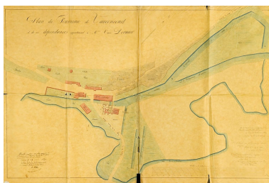
Plan du fourneau de Vauconcourt et de ses dépendances [...]. Phot. Jérôme Mongreville IVR43_20097000031NUC2A
