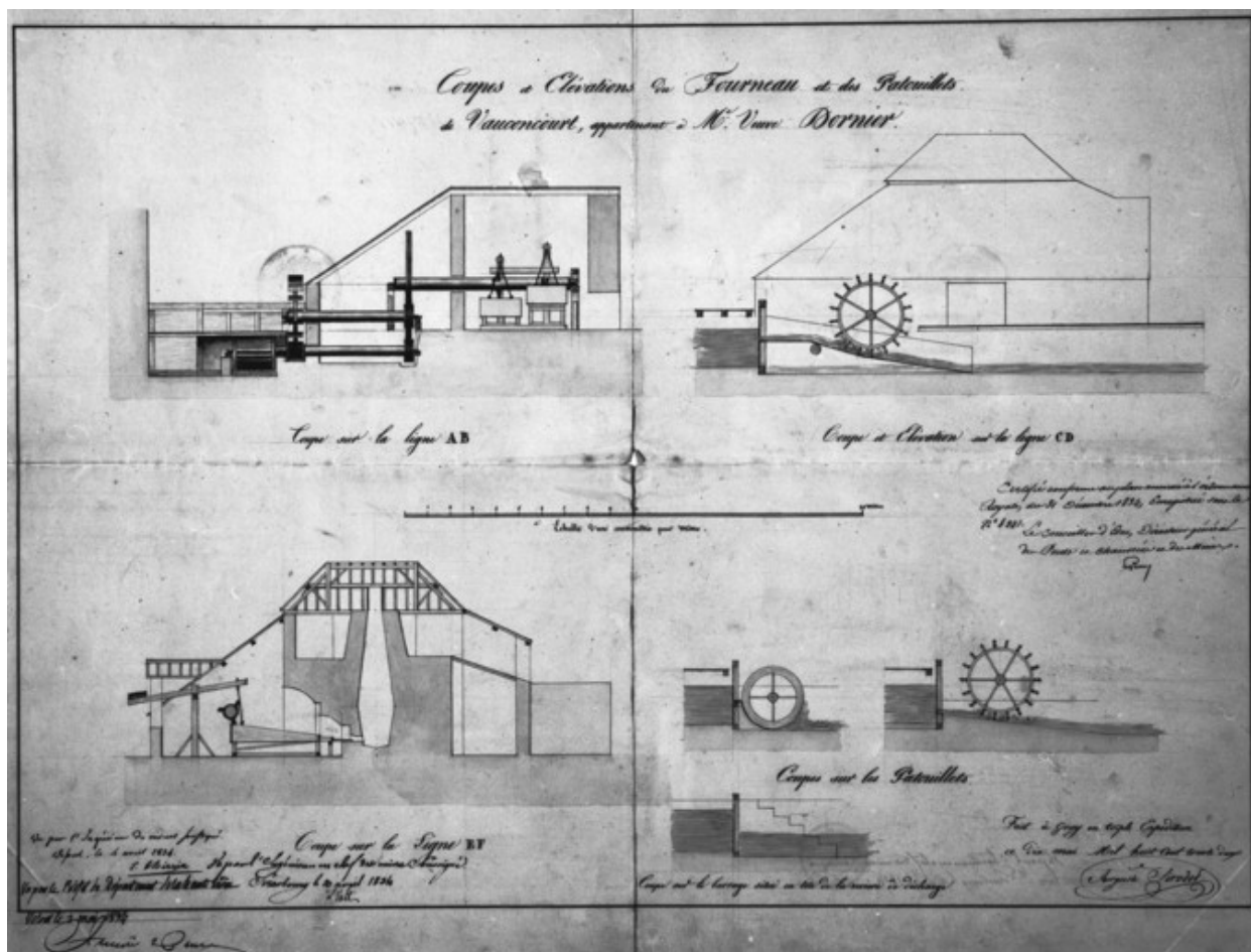
Coupes et élévations du fourneau et des patouillets de Vauconcourt, appartenant à Mme veuve Dornier.
