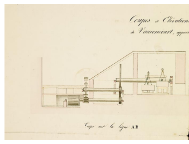
Coupes et élévations du fourneau et des patouillets de Vauconcourt [coupe transversale]. Phot. Jérôme Mongreville, Autr. Auguste Sirodot IVR43_20097000029NUC2A
