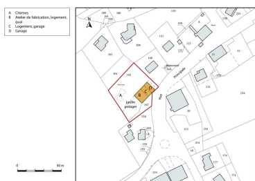
Plan-masse et de situation. Extrait du plan cadastral, 2015, section AC. Dess. Mathias Papigny IVR43_20152502292NUDA
