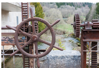
Détail du mécanisme du vannage. Phot. Jérôme Mongreville IVR43_20162500289NUC4A
