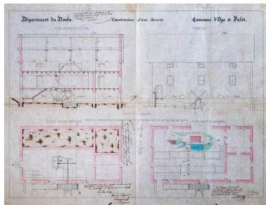
Construction d'une scierie [Plans, élévation et coupe], 1848. Phot. Jérôme Mongreville IVR43_20182500117NUC4A
