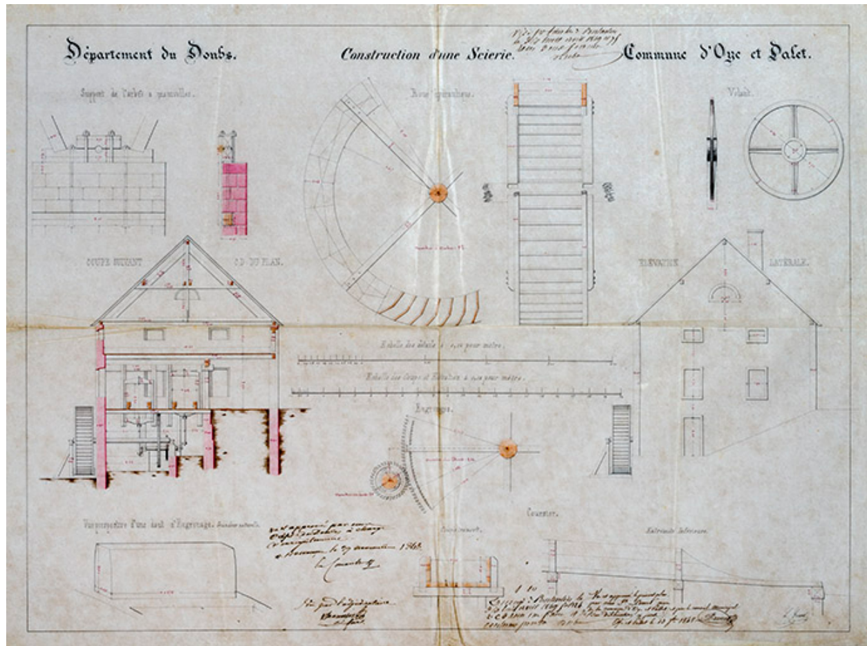
Construction d'une scierie [Elévation, coupe et détails], 1848.
