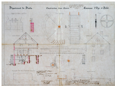
Construction d'une scierie [Elévation, coupe et détails], 1848. Phot. Jérôme Mongreville IVR43_20182500118NUC4A
