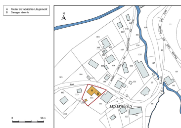
Plan-masse et de situation. Extrait du plan cadastral, 2017, section AB, 1/1 000. Dess. Mathias Papigny
