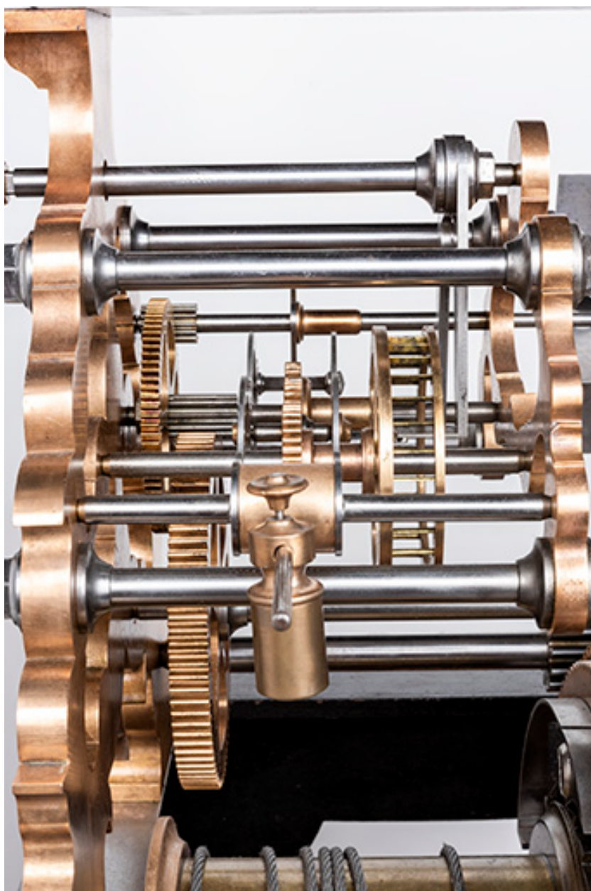
Mouvement donné en 1891 par la société Prost Frères pour l'hôtel de ville de Morez (Musée de la Lunette, Morez) : détail.
