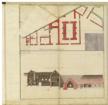
Fol. 15 Fort Saint-André-sur- Salins : plans, coupe, profil et élévation (magasin pour 60,000 milliers de poudre) - vue 3. IVR43_20243900505NUC4A
