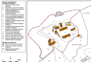
Plan-masse et de situation. Extrait du plan cadastral 2021, section I, 1/2 000. Dess. Aline Thomas IVR43_20213900168NUDA
