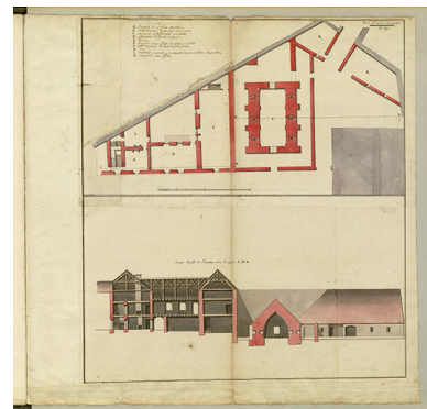
Fol. 15 Fort Saint-André-sur- Salins : plans, coupe, profil et élévation (magasin pour 60,000 milliers de poudre) - vue 1. IVR43_20243900503NUC4A
