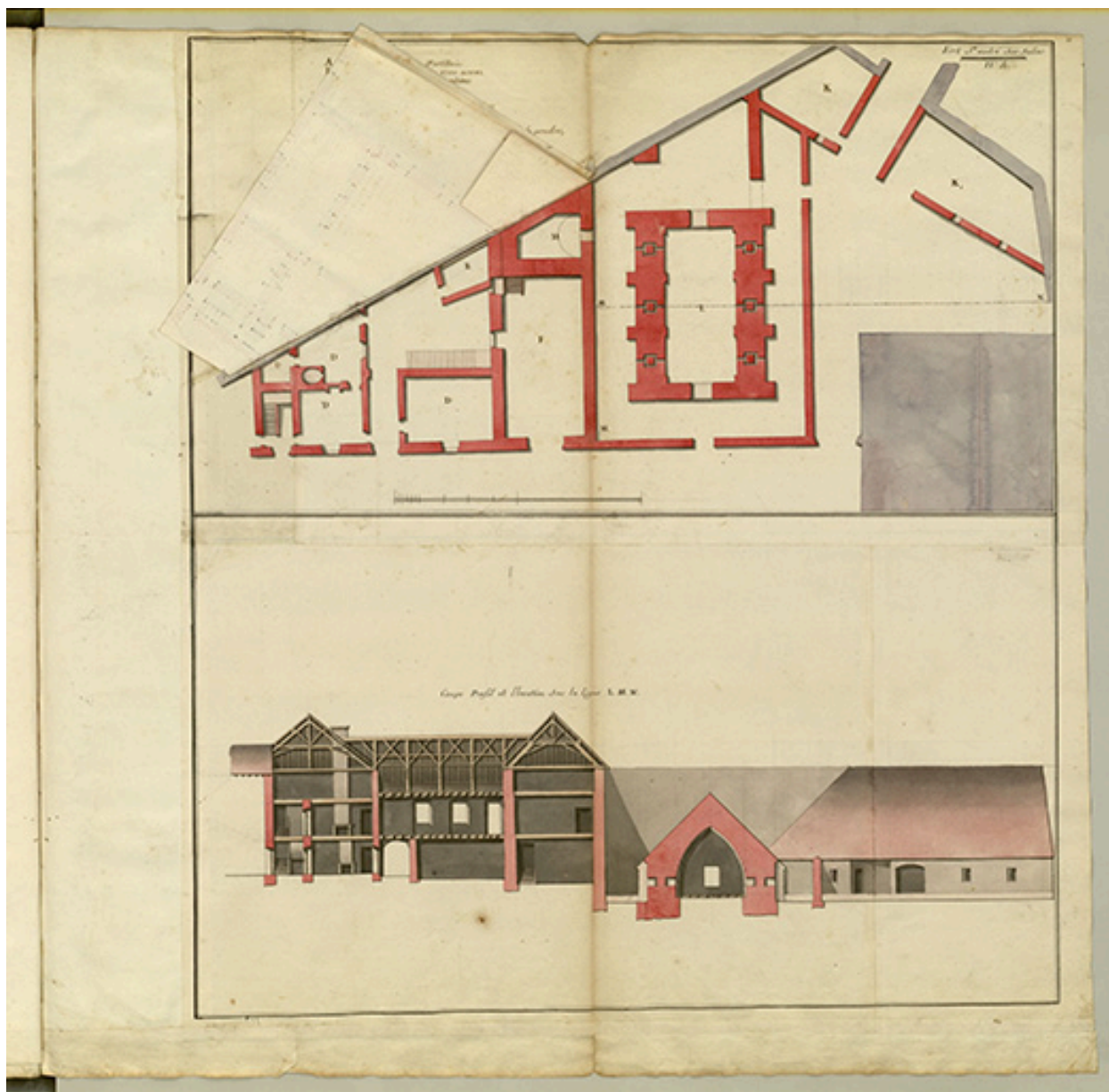
Fol. 15 Fort Saint-André-sur-Salins : plans, coupe, profil et élévation (magasin pour 60,000 milliers de poudre) - vue 3.
