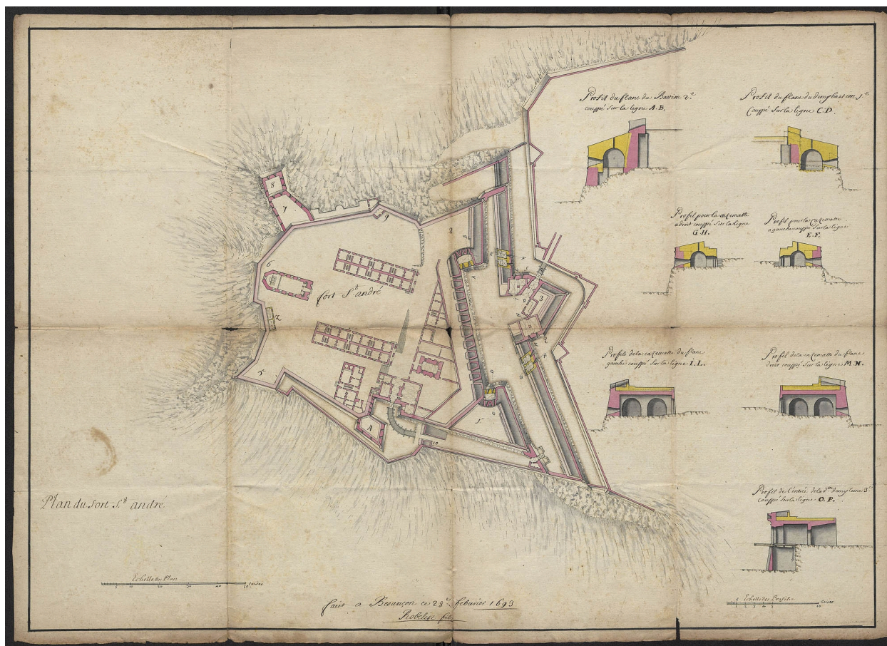
Plan du fort St-André. 28 février 1693.
