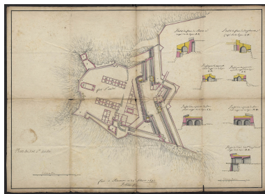
Plan du fort St- André. 28 février 1693. Autr. Isaac Robelin IVR43_20213900170NUC4A
