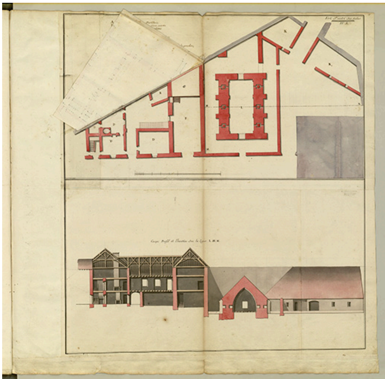
Fol. 15 Fort Saint-André-sur-Salins : plans, coupe, profil et élévation (magasin pour 60,000 milliers de poudre) - vue 2.
