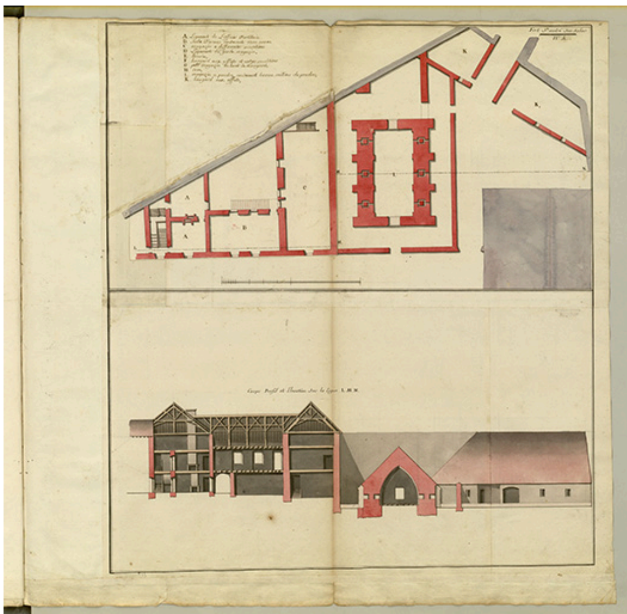
Fol. 15 Fort Saint-André-sur-Salins : plans, coupe, profil et élévation (magasin pour 60,000 milliers de poudre) - vue 1.
