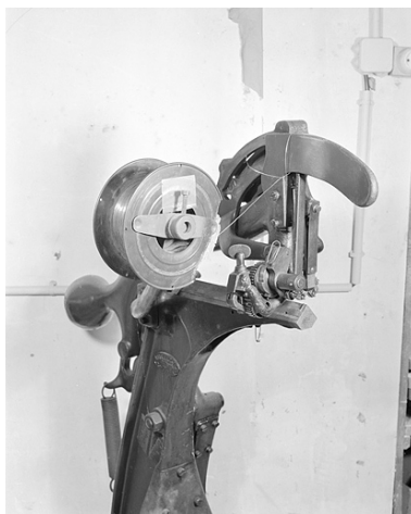
Détail du mécanisme d'agrafage. Phot. Yves Sancey IVR43_20022500762X
