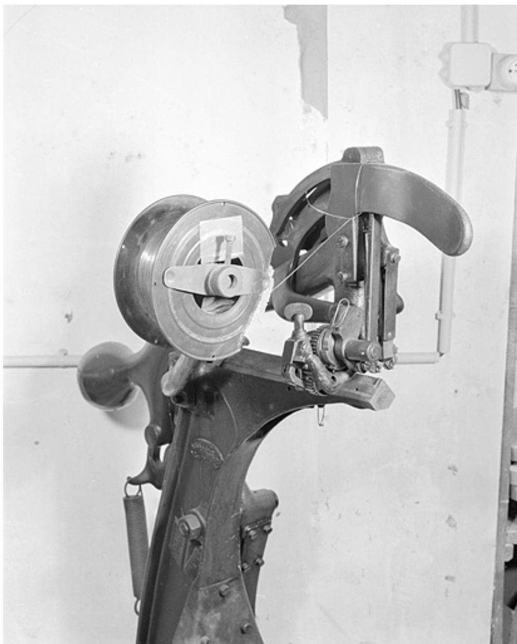
Détail du mécanisme d'agrafage.
