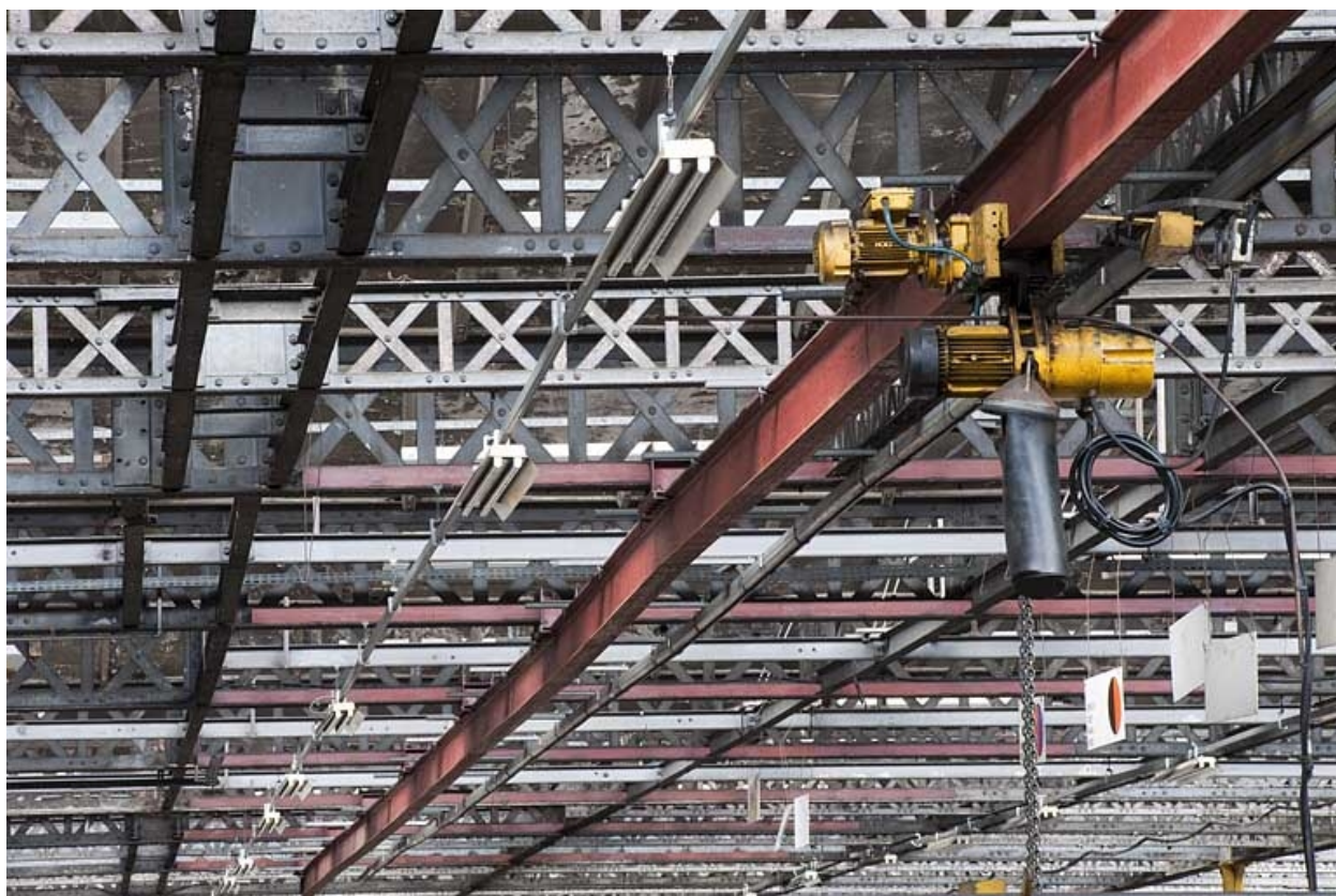
Poutrelles à treillis de la charpente.
