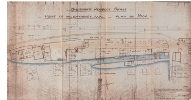
Ets Peugeot Frères. Usine de Valentigney-aval [partie nord]. Plan, échelle 1/500, s.n., 1962. Autr. IVR43_20122501690NUC2A
