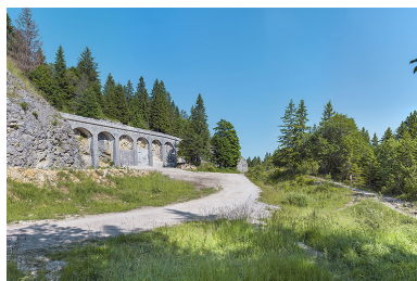
Front sud-ouest : l'enceinte close par le rempart avec ses arcs de décharge. Phot. Thierry Kuntz IVR43_20253900394NUC4A
