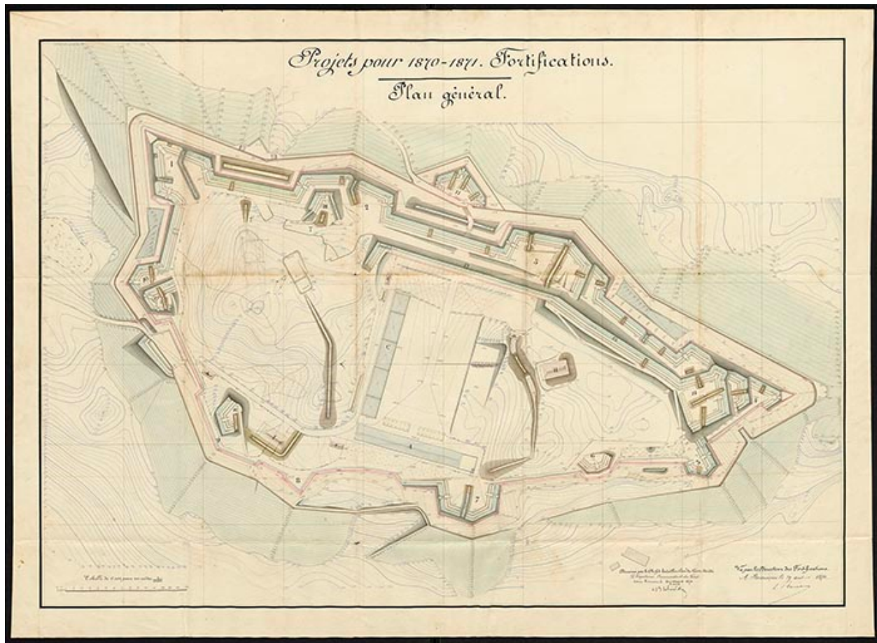
Place des Rousses - Projets pour 1870-1871 : plan général.
