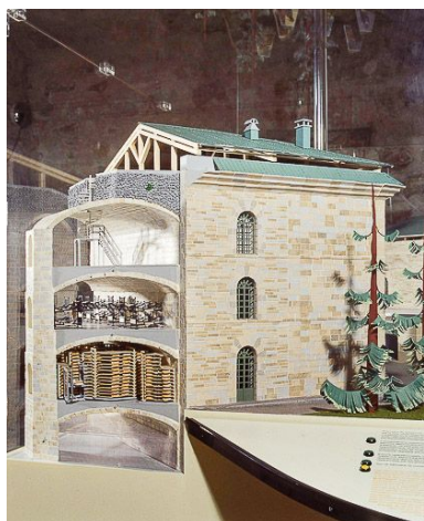
Maquette du fort, coupe sur le bâtiment Quitry et les pièces d'affinage actuelles (en 2000). Phot. Jérôme Mongreville IVR43_20003900406XA
