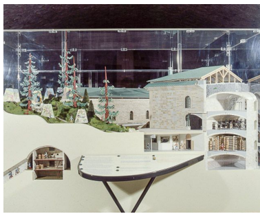
Maquette du fort, coupe sur le bâtiment Quitry et sa liaison avec le bâtiment Cavalier (en 2000). Phot. Jérôme Mongreville IVR43_20003900414XA
