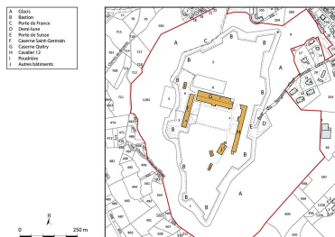
Plan masse et de situation. Extrait du plan cadastral, 2022, 1/5 000.
