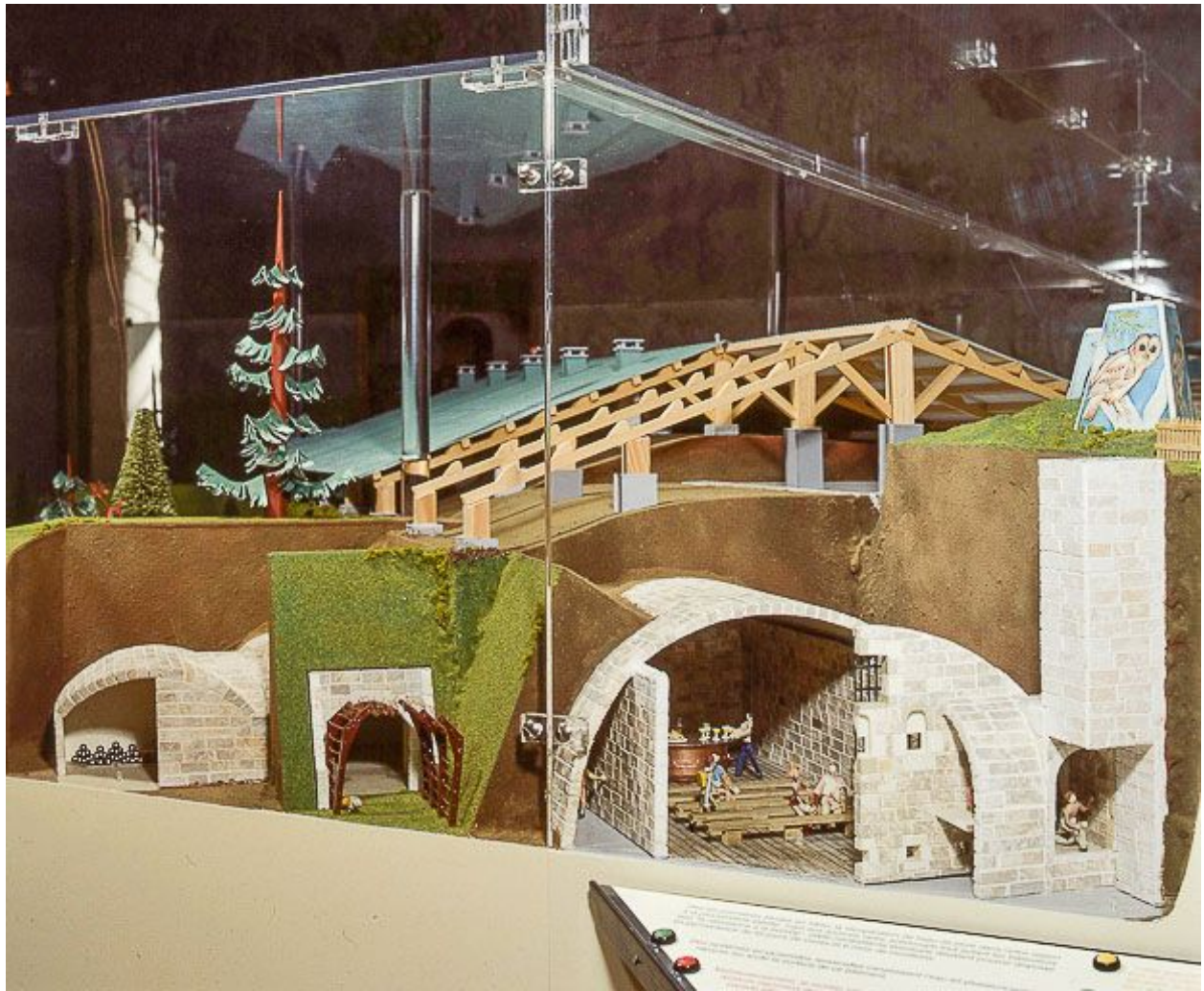
Maquette du fort, coupe sur l'ancienne poudrière (en 2000).
