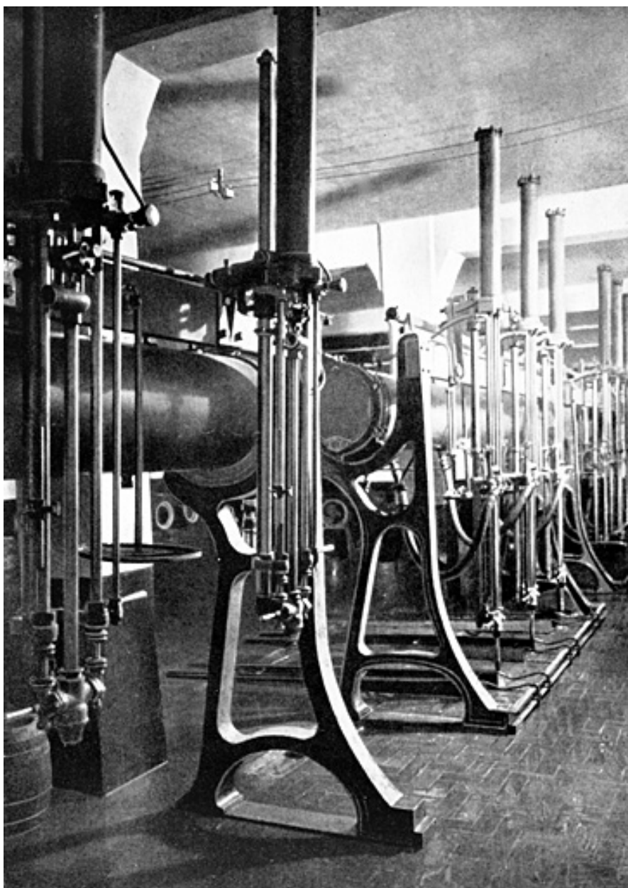
Soutireuses isobarométriques.
