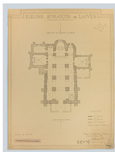
Plan de l'église relevé en 1904. Repro. Fabien Dufoulon, Phot. Renaud IVR26_20237100148NUC2A
